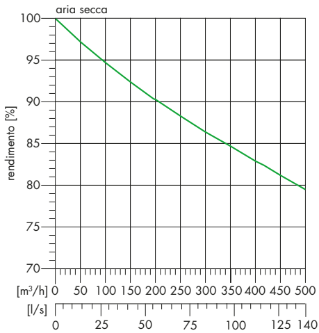
Rendimento in funzione della portata.
