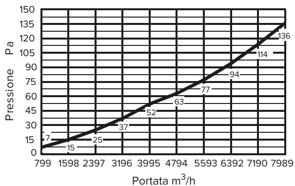
FB 6000 - F7
